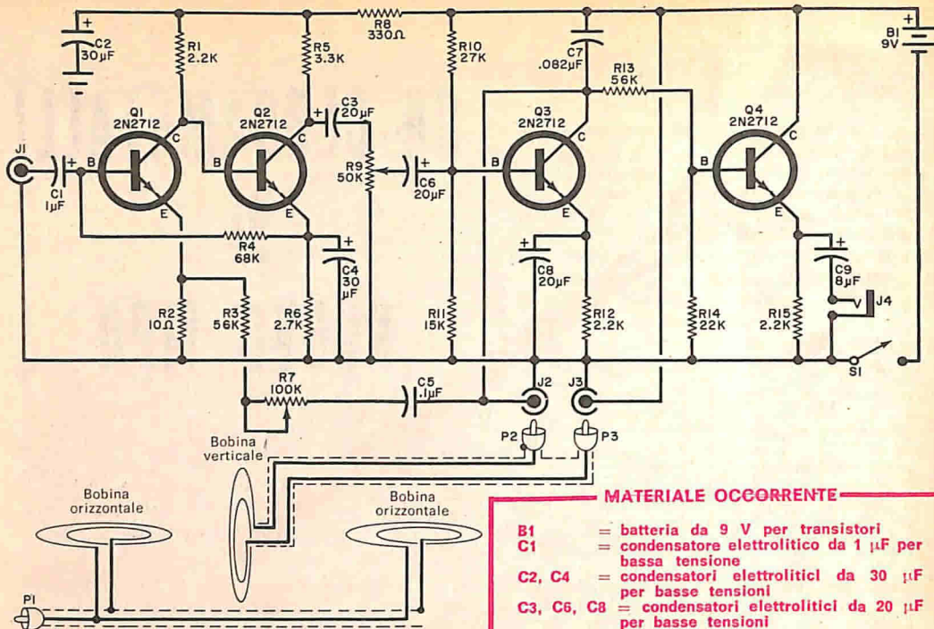
Fig. 1 - Questo circuito, che è essenzialmente un amplificatore audio instabile, entra in oscillazione quando viene rivelato un metallo tra le bobine orizzontali e quella verticale.
