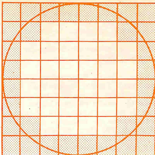
Fig. 1 - Le aree più scure di questo grafico mostrano come vengono sciupati "dadi" transistori se la basetta è rotonda anziché quadrata.
