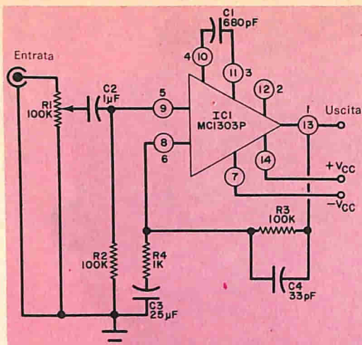
Fig. 1 - Il preamplificatore a larga banda per impieghi generici è utile per microfoni e sintonizzatori. In tutti gli schemi è rappresentata solo metà del sistema stereofonico completo.
