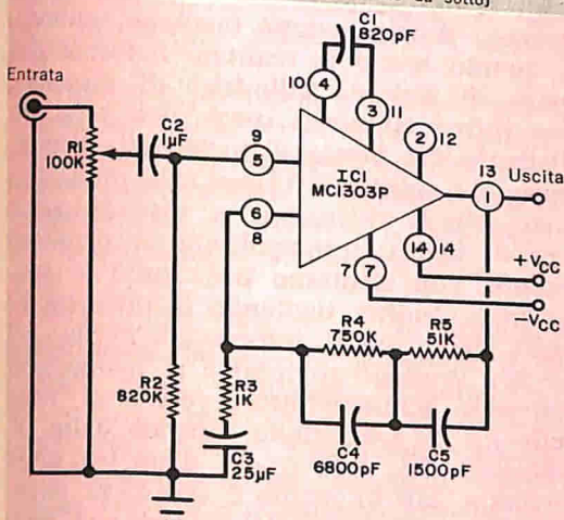
Fig. 3 - Questo circuito si usa per l'equalizzazione RIAA con giradischi a cartuccia magnetica. Per R4 si può adottare, se necessario, un valore leggermente differente (ved. testo).
