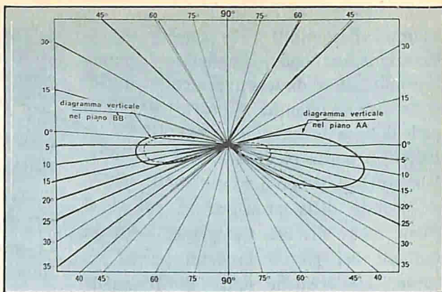
Fig. 8 - Diagramma triangolare. È simile a quello semi-circolare ma le località da servire sono poste lungo un arco maggiore di 180°. L'impianto non irradia solo in una direzione; nel diagramma verticale, l'inclinazione dei lobi è verso il basso.
