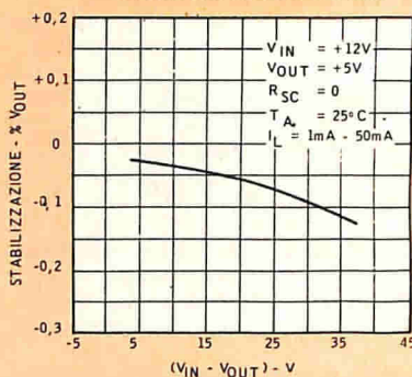
Fig. 2 - Caratteristiche di funzionamento del dispositivo L 123 della SGS.
