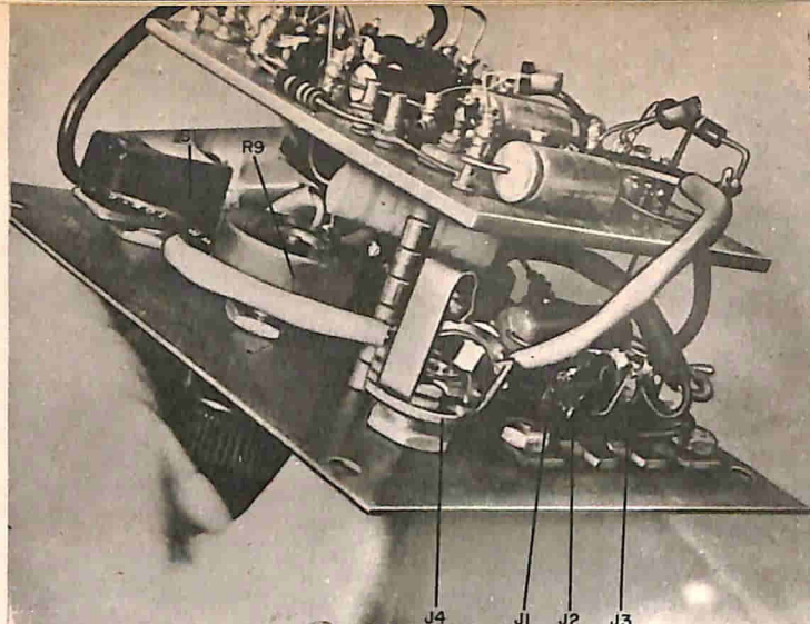
Per lasciare spazio ai componenti montati sul pannello frontale, la basetta perforata viene fissata mediante quattro distanziatori lunghi, mentre la batteria è avvitata con un fermo al pannello.
