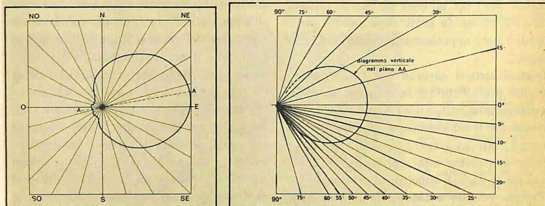
Fig. 5 - Diagramma unidirezionale limitatamente direttivo. La zona da servire è tutta compresa entro un arco di circa 90 gradi.
