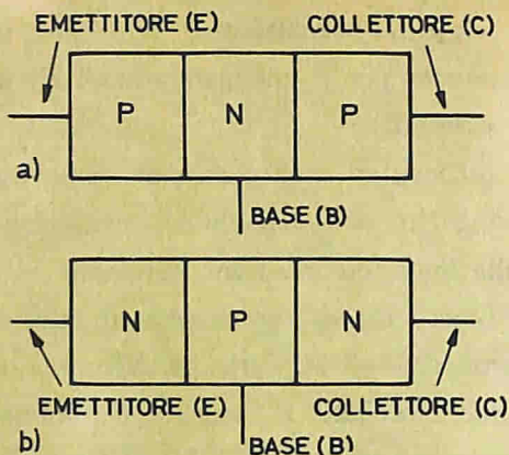
Fig. 3 - Transistori P-N-P e N-P-N rappresentati schematicamente.
