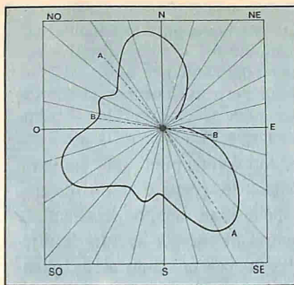
Fig. 8 - Diagramma triangolare. È simile a quello semi-circolare ma le località da servire sono poste lungo un arco maggiore di 180°. L'impianto non irradia solo in una direzione; nel diagramma verticale, l'inclinazione dei lobi è verso il basso.
