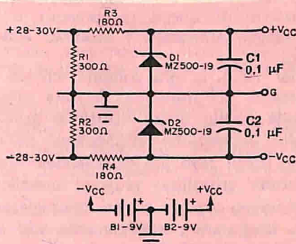
Fig. 4 - Il preamplificatore può essere alimentato sia da un circuito stabilizzato con diodi zener (in alto), sia con un paio di batterie da 9 V per radioricevitori a transistori (in basso).
