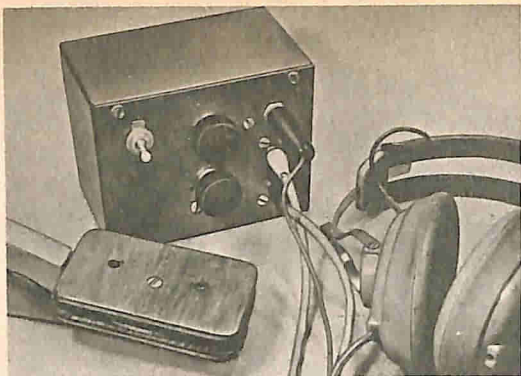
Il cercametalli è composto dalle bobine di ricerca, dalla cuffia e dalla parte elettronica.
