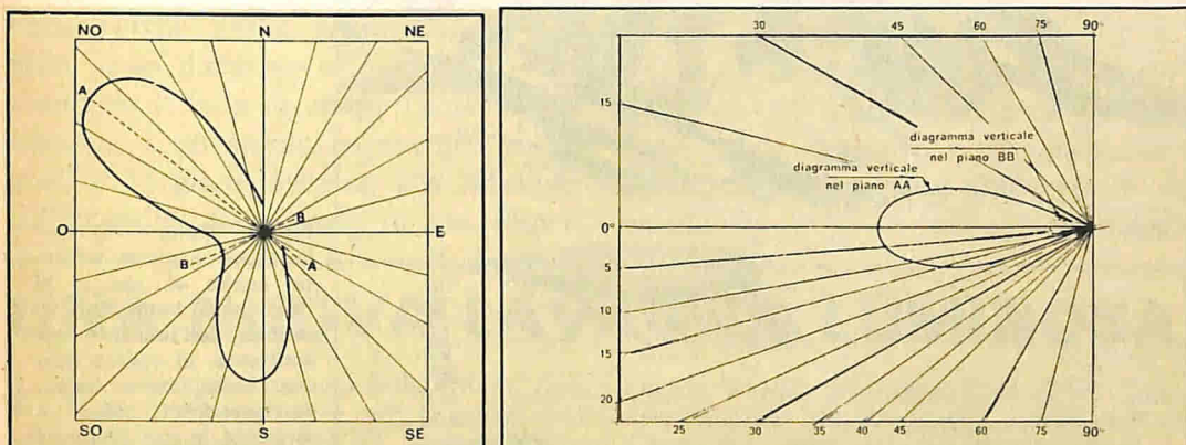
Fig. 6 - Diagramma d'irradiazione bidirezionale di accentuata direttività. Questo è il caso tipico di un impianto sistemato alla confluenza di due vallate.
