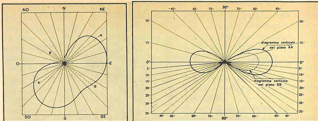
Fig. 4 - Diagramma d'irradiazione semi-circolare. L'energia viene irradiata prevalentemente lungo un arco di circa 180 gradi. È il caso tipico di un impianto posto sul versante montano che delimita una zona pianeggiante.
