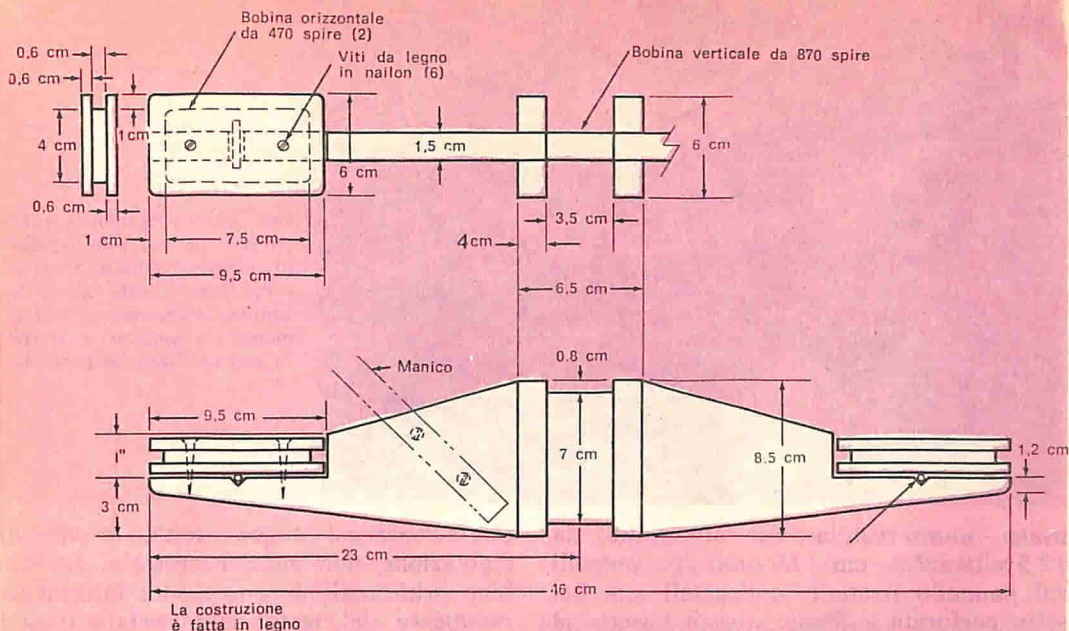
Fig. 2 - Ad eccezione del filo delle bobine, nella costruzione della testata di ricerca non vengono usati metalli. Le bobine orizzontali sono fissate con viti di nailon; il resto è incollato con colla forte.
