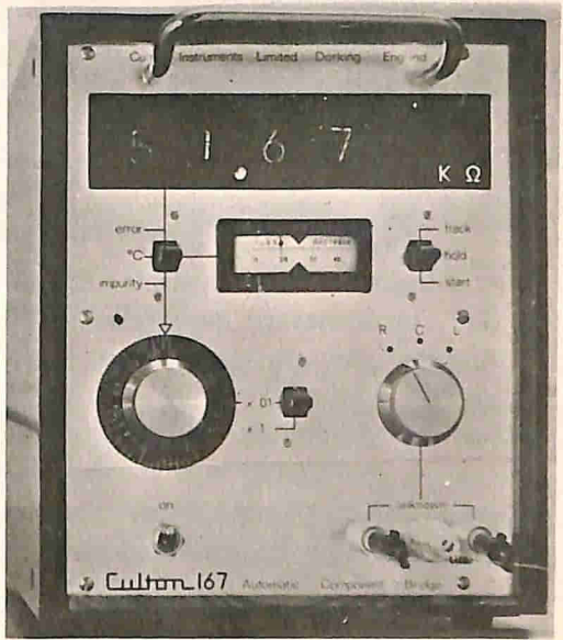
Fig. 1 - Ponte di misura automatico Cultron.
