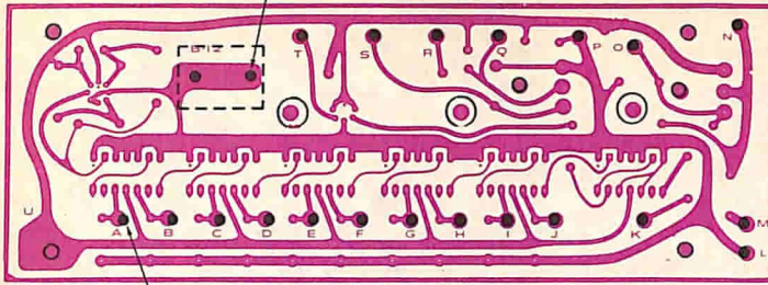
Fig. 3 - Piano di foratura del circuito stampato; nei tre fori più grandi si montano i distanziatori per i condensatori di filtro. L'impiego di venti cilindretti di ancoraggio è del tutto facoltativo.
