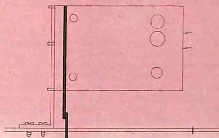
Sistema di fissaggio su circuito stampato (a) e con piastra metallica (b).
