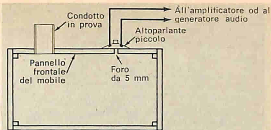
Fig. 3 - Per accordare un mobile, fissate un altoparlante sopra un foro di piccole dimensioni, e poi variate la lunghezza del condotto di cartone.
