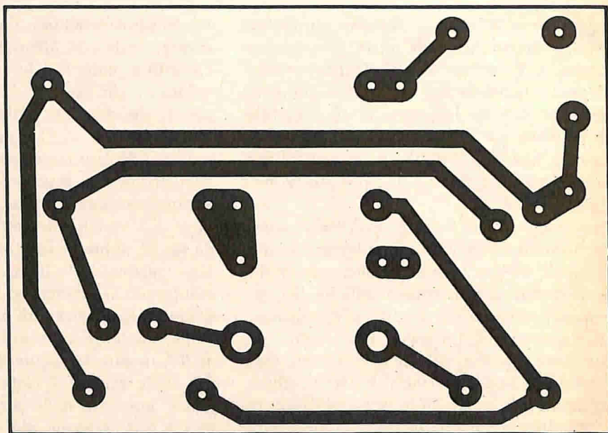
Fig. 2 - Circuito stampato in grandezza naturale. La disposizione delle parti si può vedere nella foto qui in alto e nella fig. 3. Il diametro dei fori più grandi deve essere adatto al diametro dei terminali dello strumento usato. Alcuni strumenti hanno i terminali di diametro uguale a quello dei fori della figura, altri presentano fori più grandi.
