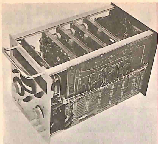
Fig. 3 - Interno del ponte di misura, da cui sono visibili i circuiti stampati montati verticalmente.
