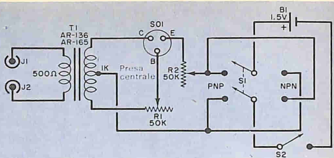
Fig. 2 - Il circuito di questo prova-transistori è essenzialmente un oscillatore Hartley modificato. Può controllare guadagni ridotti e scartare transistori n-p-n e p-n-p in cortocircuito, interrotti, con perdite eccessive o guadagno troppo basso.
