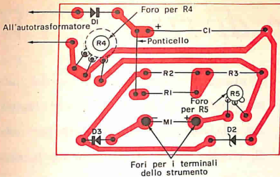
Fig. 3 - Disposizione dei componenti sul circuito stampato; come si può rilevare chiaramente, un ponticello collega R1 al terminale positivo di C1. I fori per i terminali dello strumento e per il potenziometro devono essere larghi appena quanto occorre per consentire un montaggio stretto.
