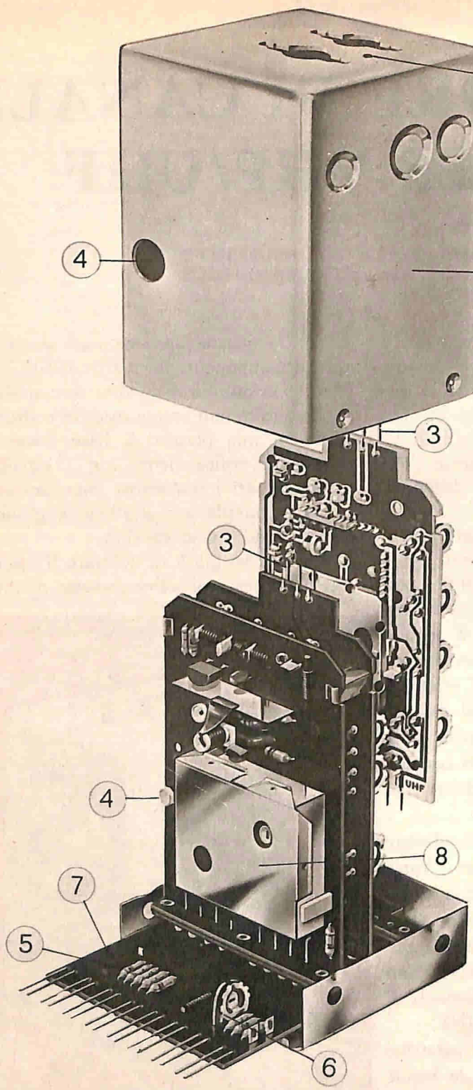
Vista interna del selettore di canali VHF-UHF della Philips.
