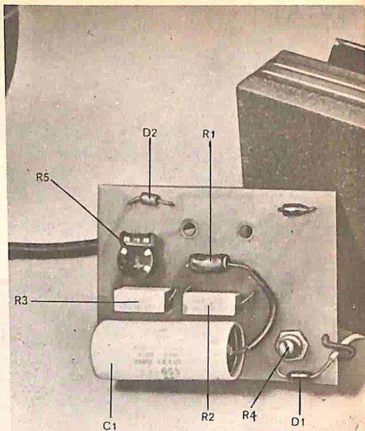
Tutti i componenti si devono montare sul circuito stampato, il quale viene poi fissato allo strumento usando le viti dei suoi terminali.
