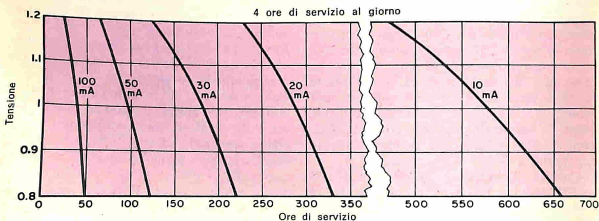
Fig. 3 - Il grafico indica le ore approssimate di servizio che una certa pila da 1,5 V può fornire usandola quattro ore al giorno. La durata di una batteria dipende però da molti fattori, tra cui la temperatura, la corrente richiesta e la tensione finale sufficiente. Si noti che le ore di servizio previste crescono diminuendo la corrente di scarica, il che vale anche per gli amper-ora. Al livello di 0,8 V ad un carico di 100 mA (prima curva a sinistra) corrispondono circa 5 amper-ora. Con un carico di 10 mA (ultima curva a destra) si ottiene invece una capacità di circa 6,6 amper-ora.
