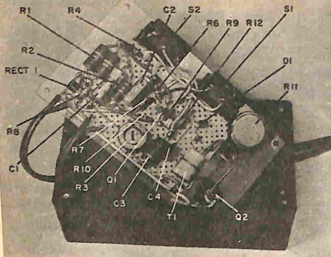
Fig. 3 - Come si può rilevare da questa figura, la disposizione delle parti non è critica; occorre però fare attenzione ad isolare il transistor Q2 dal pannello.
