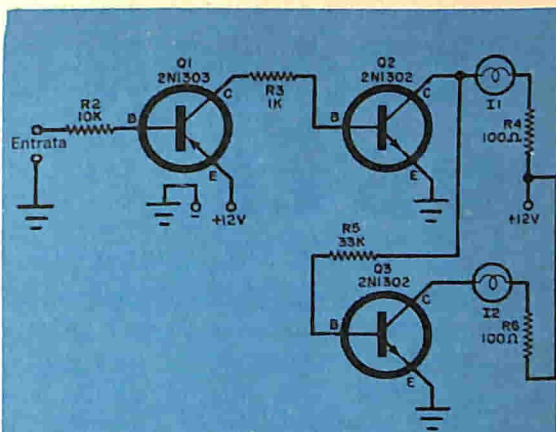
Fig. 4 - L'indicatore a flip-flop è sicuro in quanto indica che il circuito controllato funziona. Quando I1 è accesa, I2 è spenta e viceversa. Volendo, si può aggiungere il circuito della figura 3.
