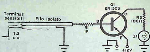
Fig. 2 - Il circuito indicatore ad autoagganciamento mantiene accesa la lampadina anche quando il segnale eccitatore è cessato. La lampadina I1, in serie con il resistore da 100 Ω, può essere collegata in parallelo alla lampadina I2 e al resistore R2.
