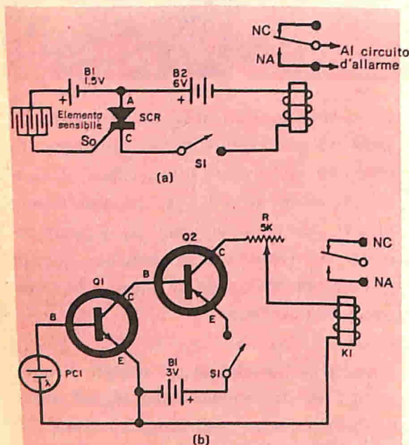
Fig. 2 - Schemi di due circuiti di controllo: (a) rivelatore di pioggia con raddrizzatore controllato al silicio a bassa tensione; (b) commutatore a due transistori, che funziona solo quando l'elemento sensibile (PC1) viene illuminato.
