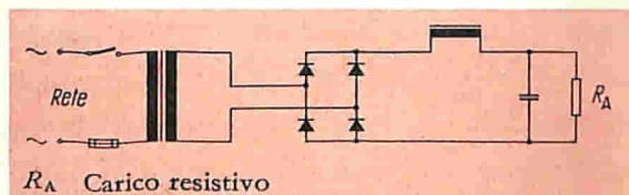
Fig. 3 - Disinserzione dei collegamenti di un trasformatore sull'avvolgimento primario.
