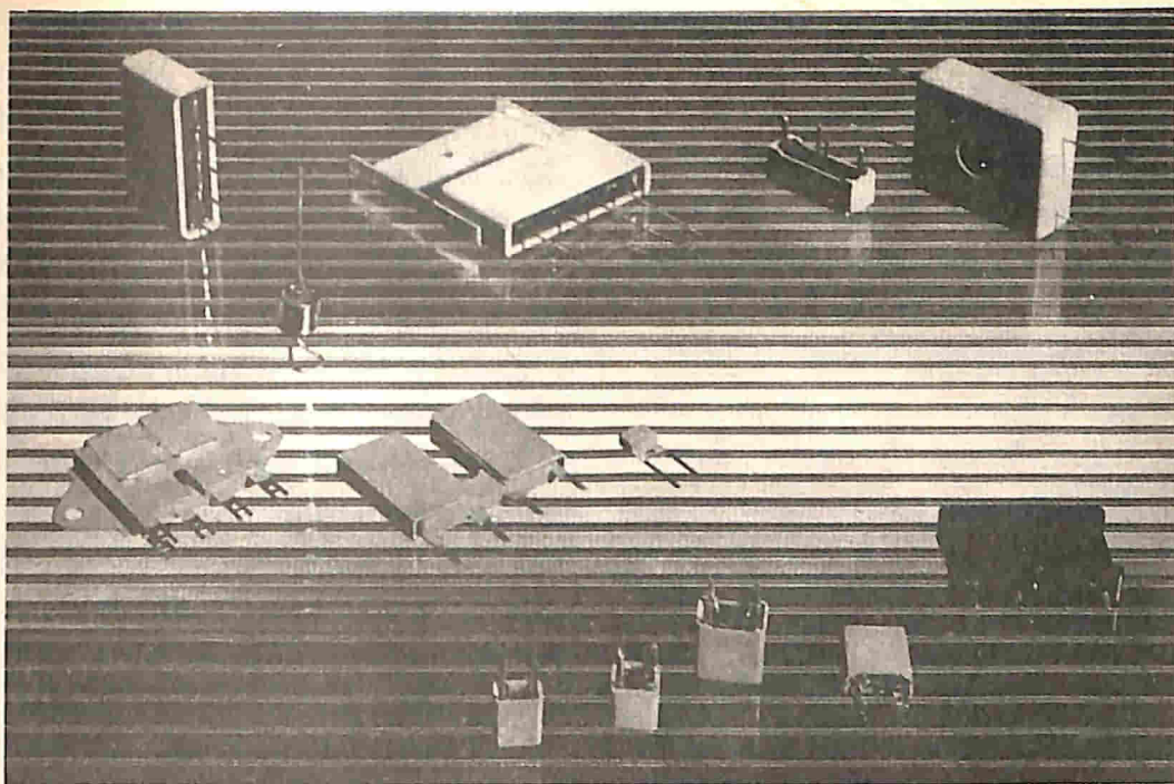
Fig. 1 - Esempi di alcuni nuovi modelli di microraddrizzatori al selenio ed al silicio. In prima fila si vedono microraddrizzatori al selenio, nella fila di mezzo raddrizzatori al selenio aggraffati mentre nella terza fila sono illustrati microraddrizzatori al silicio.
