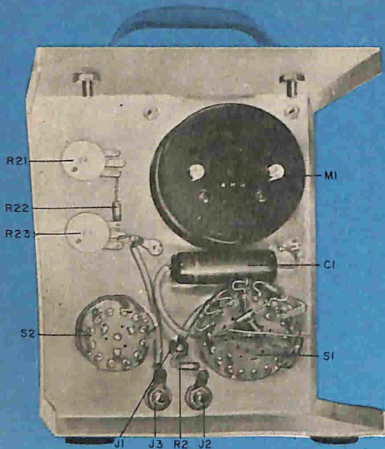
In queste illustrazioni si vede il pannello frontale (a sinistra) su cui sono montati alcuni componenti ed il telaio di materiale isolante (a destra) sul quale sono state fissate le altre parti.
