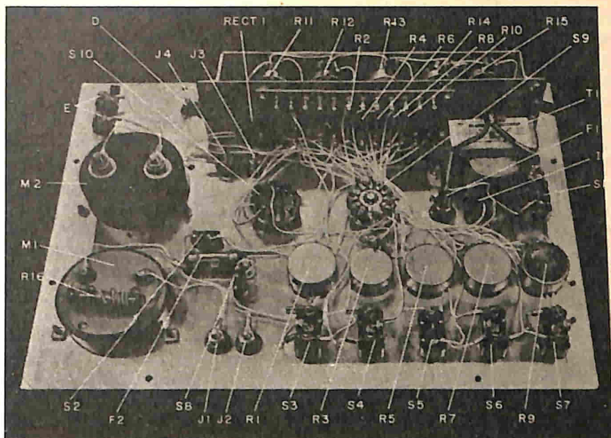
Fig. 2 - L'intero montaggio si effettua sul pannello frontale. La costruzione del dispositivo non è però così complicata come sembra e la disposizione delle parti non è critica. Si faccia attenzione alla polarità del raddrizzatore, e si tenga presente che è meglio completare il montaggio ed effettuare tutti i collegamenti prima di procedere alla installazione dei due strumenti.
