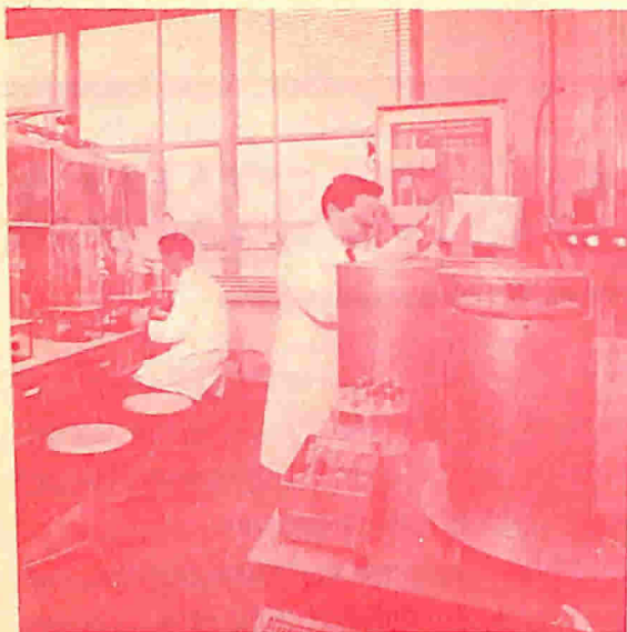
Fig. 2 - In questo angolo del reparto della fabbrica Philips di Monza, in cui si costruiscono i tubi ad onde progressive, si scorgono alcune apparecchiature per le saldature vetro-metallo e ceramica-vetro per tenute ad altissimo vuoto. (documentazione Philips)
