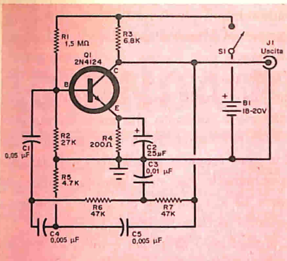
Fig. 3 - Oscillatore audio a doppio T da 1 kHz, progettato dalla Motorola, il quale può essere usato in tutte le applicazioni in cui è necessario un segnale sinusoidale di frequenza fissa.
