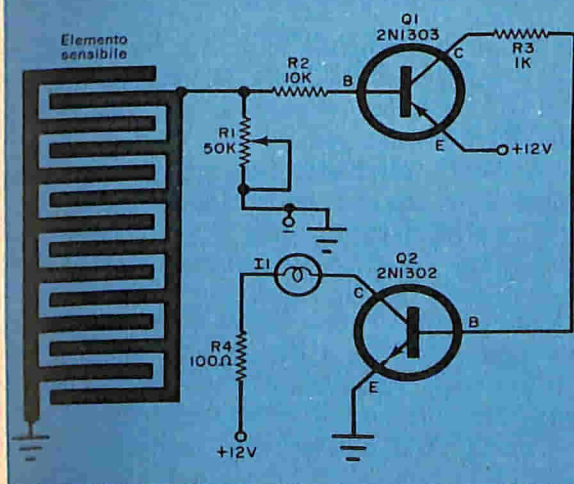
Fig. 3 - La sensibilità può essere aumentata regolando la polarizzazione appena al di sotto del punto di conduzione di Q1. Qualsiasi ulteriore diminuzione della resistenza causata, per esempio, da umidità tra gli elettrodi dell'elemento sensibile, farà condurre Q1 e Q2 ed accendere I1.
