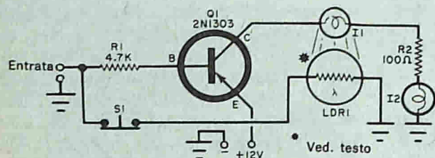
Fig. 2 - Il circuito indicatore ad autoagganciamento mantiene accesa la lampadina anche quando il segnale eccitatore è cessato. La lampadina I1, in serie con il resistore da 100 Ω, può essere collegata in parallelo alla lampadina I2 e al resistore R2.
