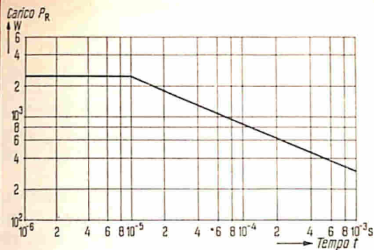
Fig. 4 - Grafico della potenza di un raddrizzatore insensibile ad impulsi di tensione inversa, espressa in funzione della durata t dell'impulso.
