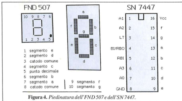
Figura 4. Piedinatura dell'FND 507 e dell'SN 7447.
