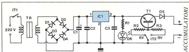
Figura 1. Lo schema elettrico rivela l'impiego di un circuito integrato regolatore.
