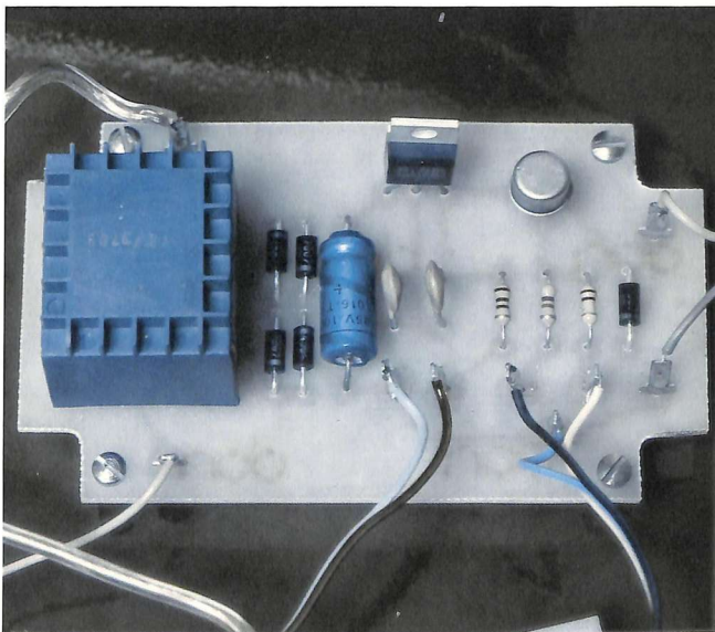
Foto 2. Un modulo molto semplice da realizzare.
