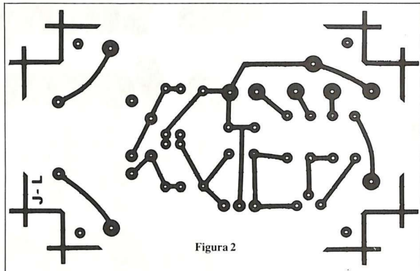
Figure 2 e 3. Il tracciato del circuito stampato è facile da riprodurre con l'impiego di trasferibili.
