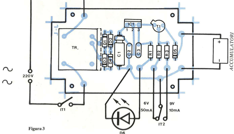
Figure 2 e 3. Il tracciato del circuito stampato è facile da riprodurre con l'impiego di trasferibili.
