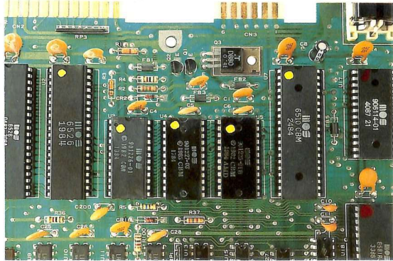
Figura 1a. Le tre ROM presenti nel C64.
