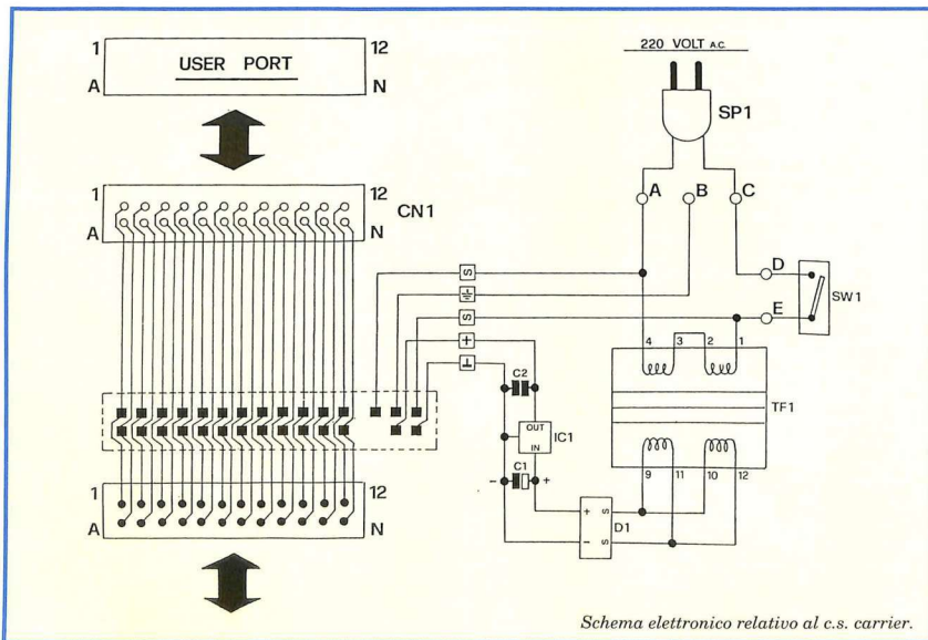
Schema elettronico relativo al c.s. carrier.
