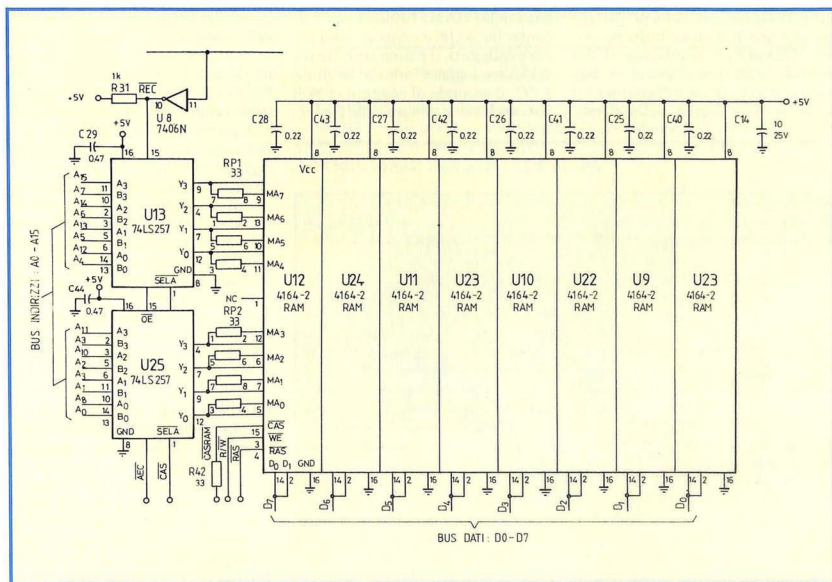
Figura 2b. Lo schema elettrico della memoria RAM.
