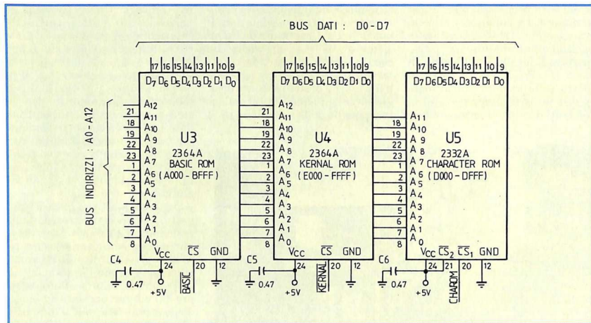
Figura 1b. Ecco tutti i collegamenti delle tre ROM.
