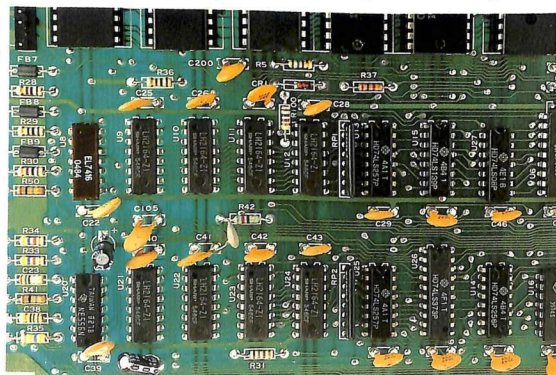
Figura 2a. La memoria ROM del C64.
