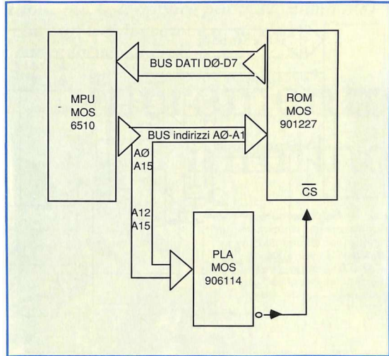
Figura 4. Schema del principio dell'operazione di lettura di una ROM.
