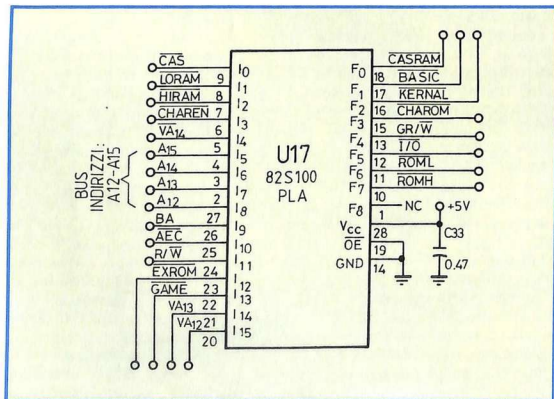
Figura 3. Le connessioni elettriche del PLA.
