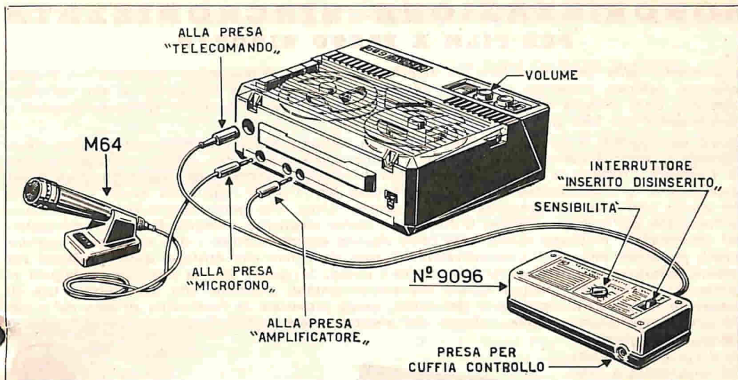
Collegamento del « Vocemagic » 9096 al G 681.
