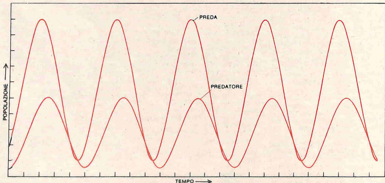
FIG. 1 Una relazione teorica predatore-preda: una soluzione alle equazioni di Lotke-Volterra
