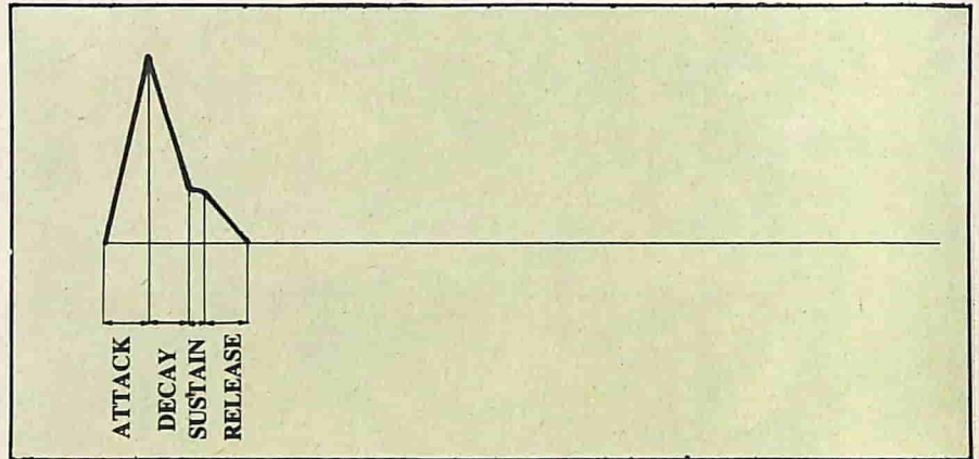
Figura 8: involuppo del suono emesso da un tamburo.
