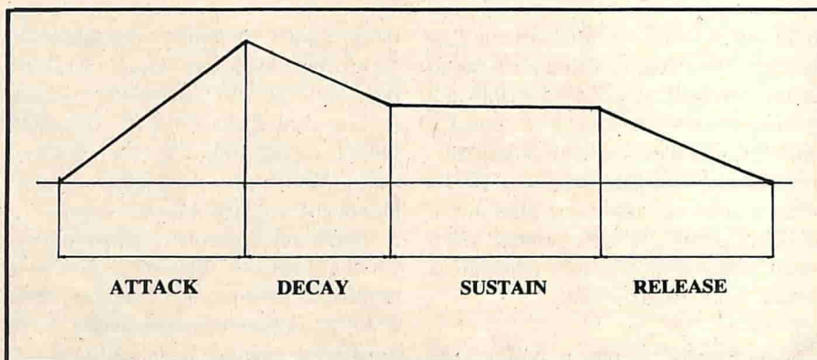
Figura 7: inviluppo del suono.
