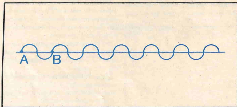
Figura 5: rappresentazione grafica della seconda armonica superiore.
