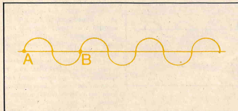
Figura 4: rappresentazione grafica della prima armonica superiore.
