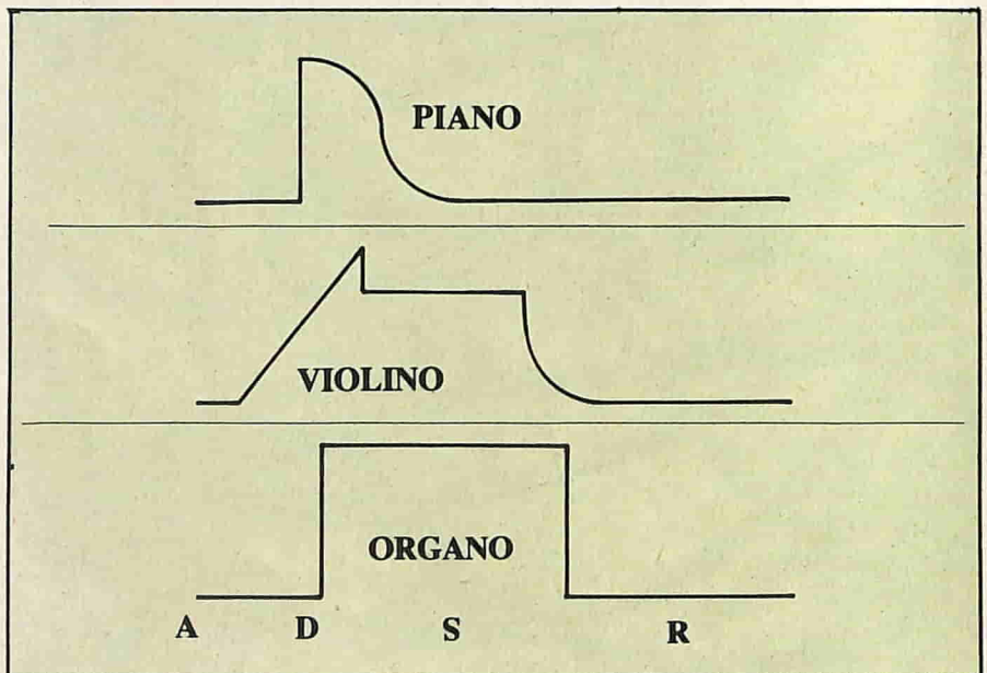
Figura 9: involuppo del suono emesso da strumenti musicali.
