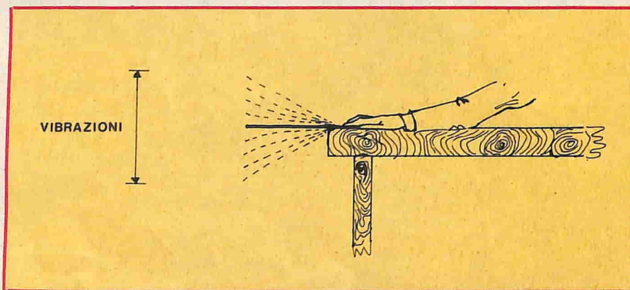
Figura 1: una lamina colpita compie vibrazioni.
