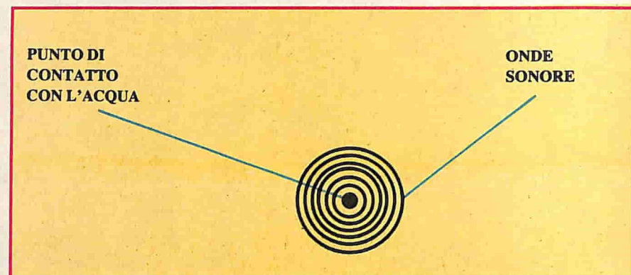
Figura 2: onde provocate dalla caduta di un sasso in uno stagno.
